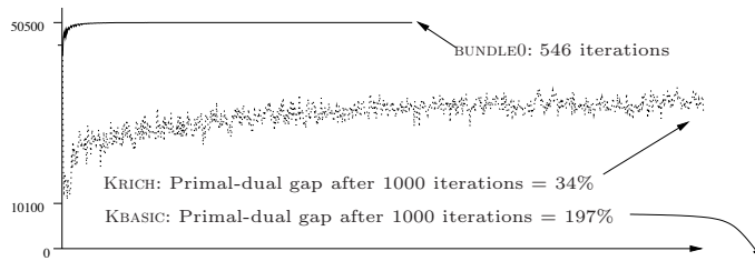
Fig. 2.5. TSP: Kelley vs. bundle on pcb442
