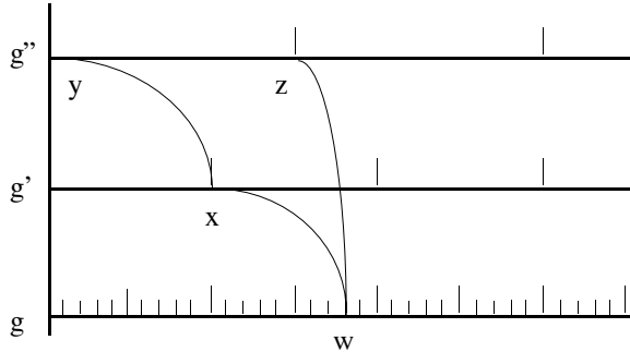
Figure 5. En cas de décalage des échelles (c'est-à-dire qu'à une graduation de la granularité supérieure ne corresponde pas de graduation de la granularité inférieure), la propriété de transitivité cumulée n'est pas vérifiée:
